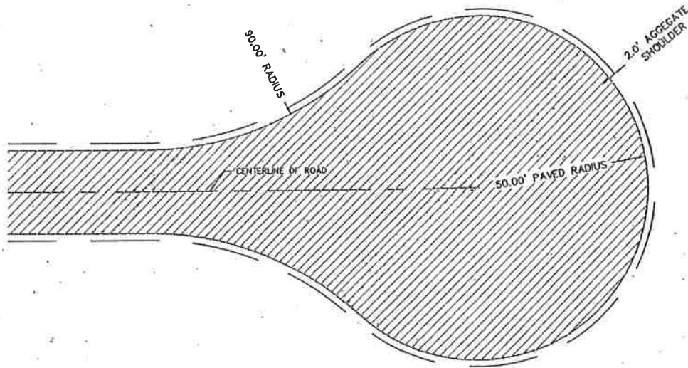
CUL-DE-SAC
