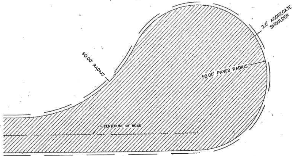
OFFSET CUL-DE-SAC
